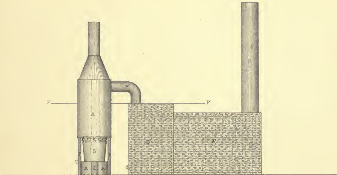
Fig. 1 SIDE ELEVATION
