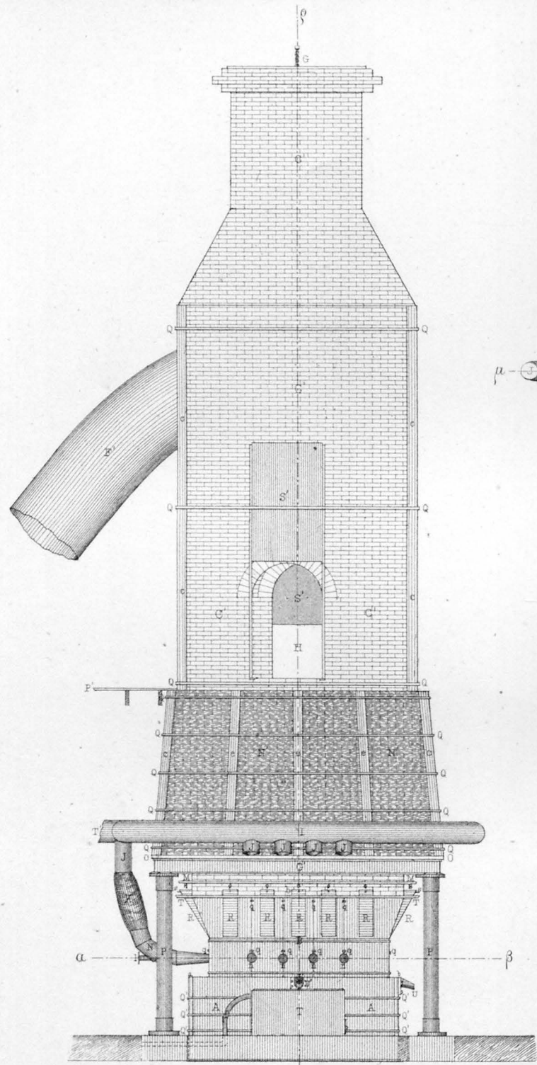
Fig. 1 ELEVATION
